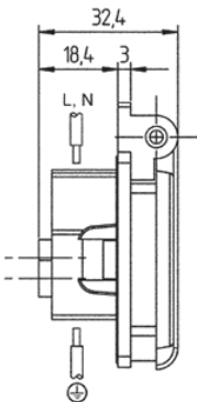
图纸 1 MB 584 尺寸毫米
