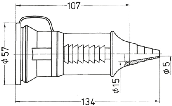
图纸 3 MB 39 尺寸毫米
