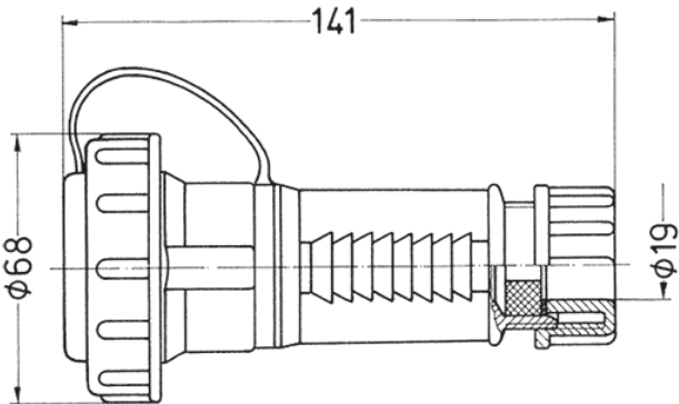
图纸 3 MB 41 尺寸毫米
