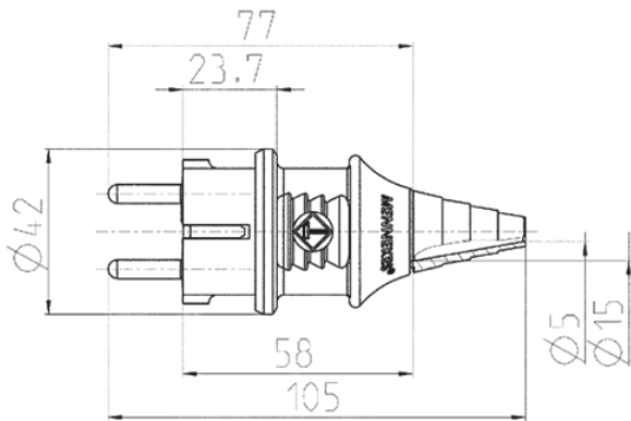
图纸 2 MB 139 尺寸毫米
