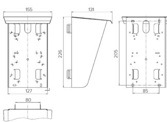
图纸 1 MB 431 尺寸毫米
