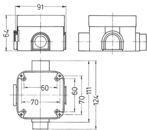
图纸 1 MB 334 尺寸毫米
