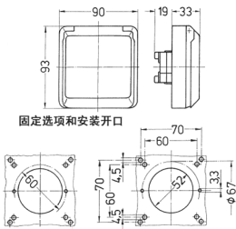
图纸 1 MB 304 尺寸毫米
