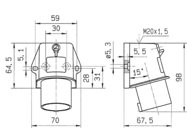
图纸 2 MB 213 尺寸毫米
