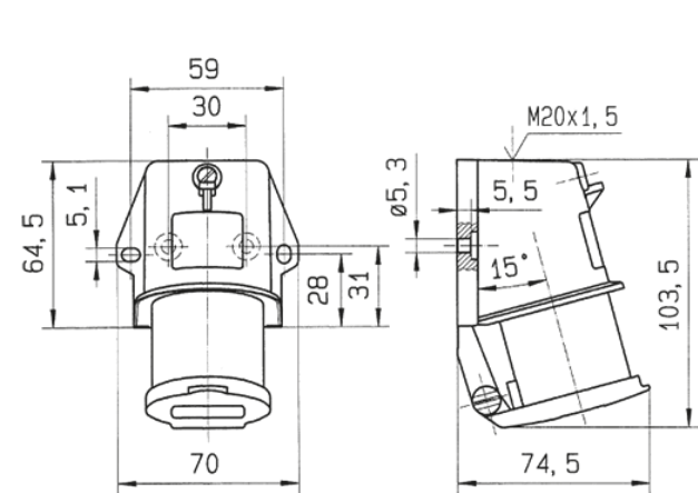
图纸 2 MB 212 尺寸毫米
